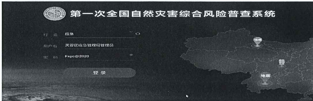
图 1 登陆系统
